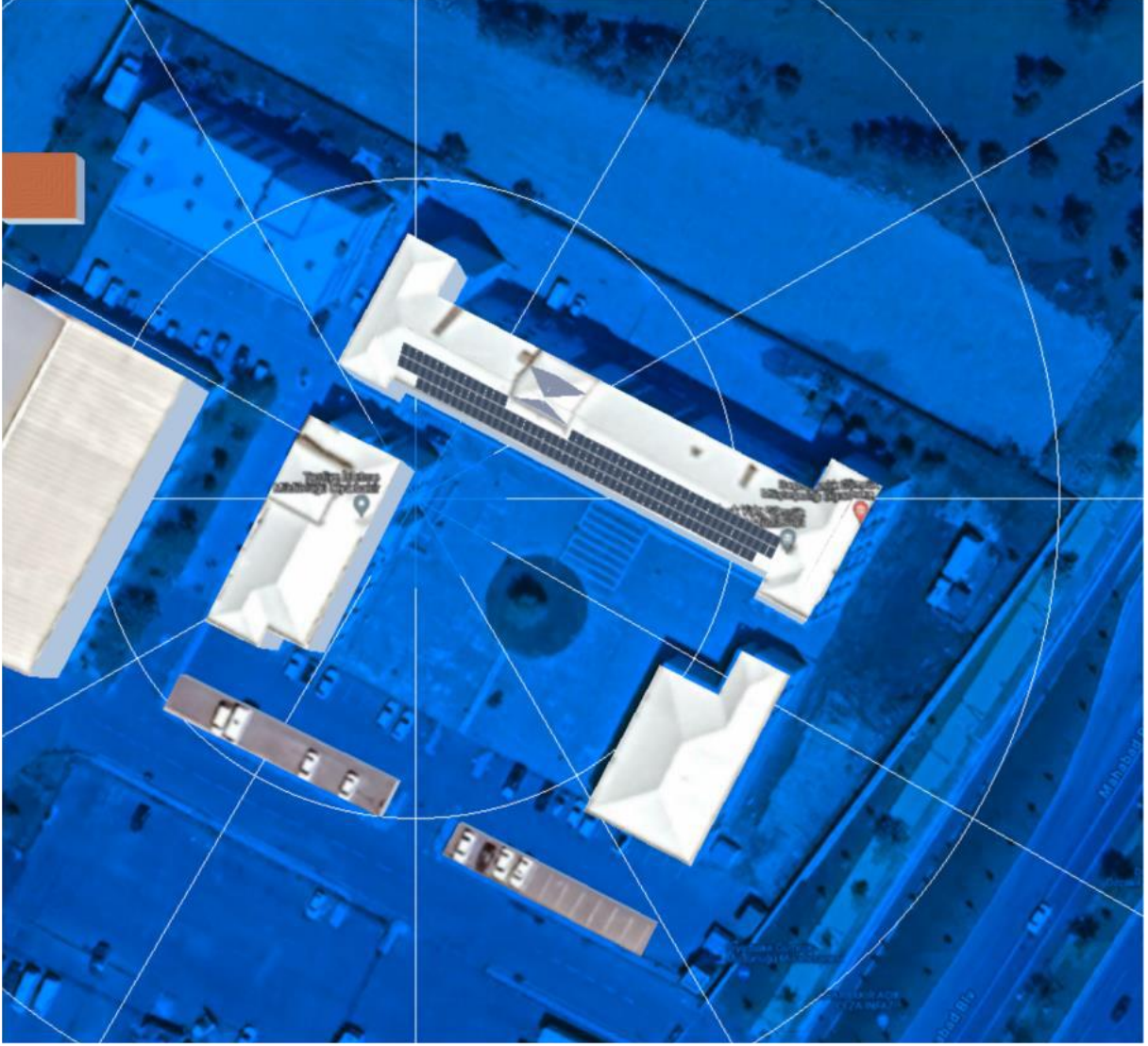
Şekil 5: Diyarbakır Gümrük Müdürlüğü Ana Bina Çatı Üstü 82,50 kWp PV Kurulum Tasarım Görünümü
