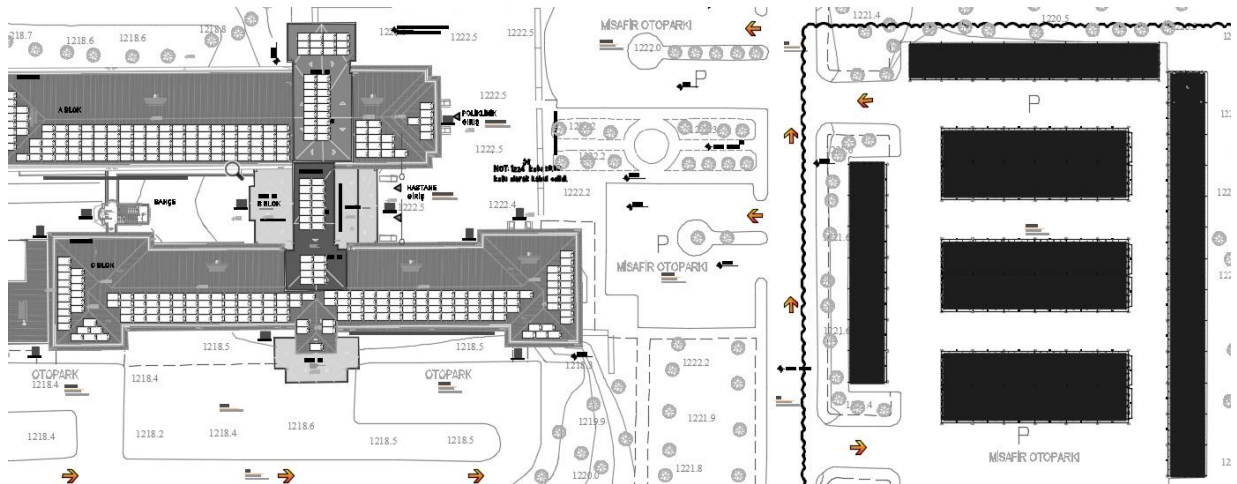
Şekil 6 Beytepe Şehit Murat Erdi Eker Devlet Hastanesi Çatı ve Otopark GES Tesisatı Yerleşimi
