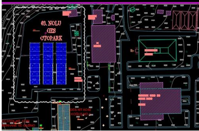
Şekil 10. Ankara Jandarma Sahil Güvenlik Akademisi GES-3 Sistemi Yerleşim Planı
