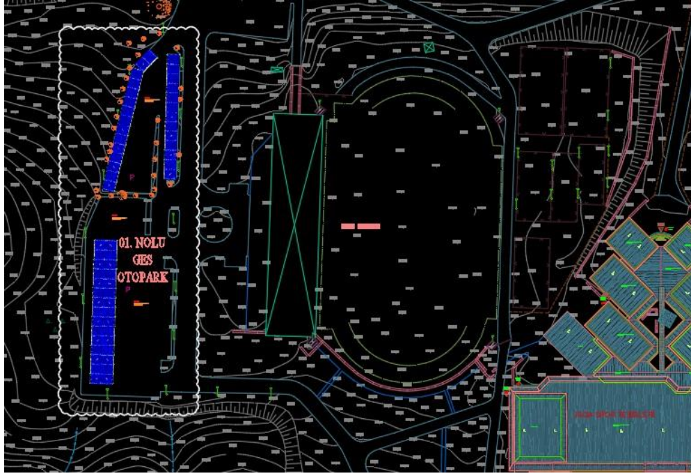
Şekil 8. Ankara Jandarma Sahil Güvenlik Akademisi GES-1 Sistemi Yerleşim Planı
