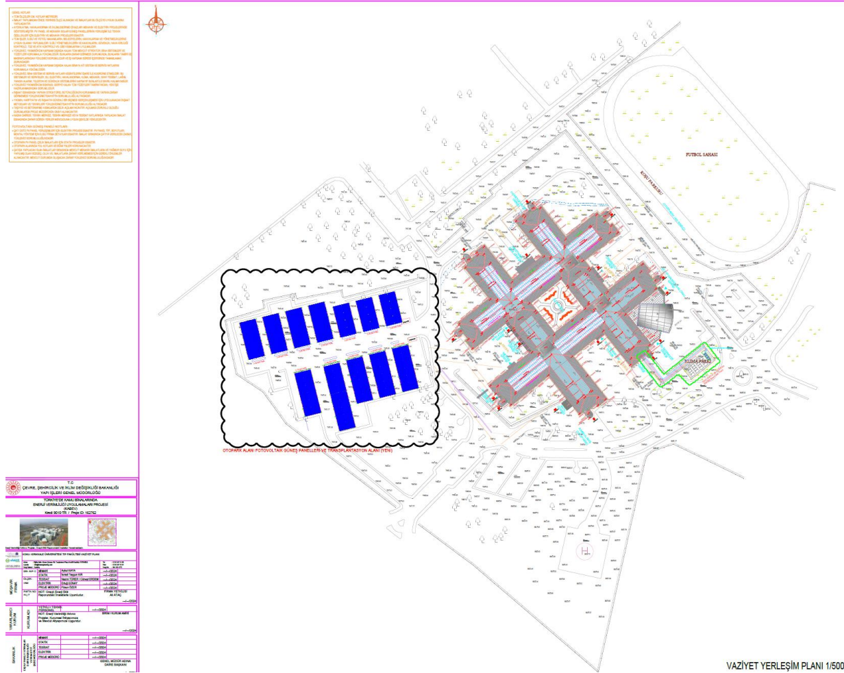
Şekil 4 Kırıkkale Üniversitesi Tıp Fakültesi ve Hastanesi GES Sistemi Yerleşim Planı
