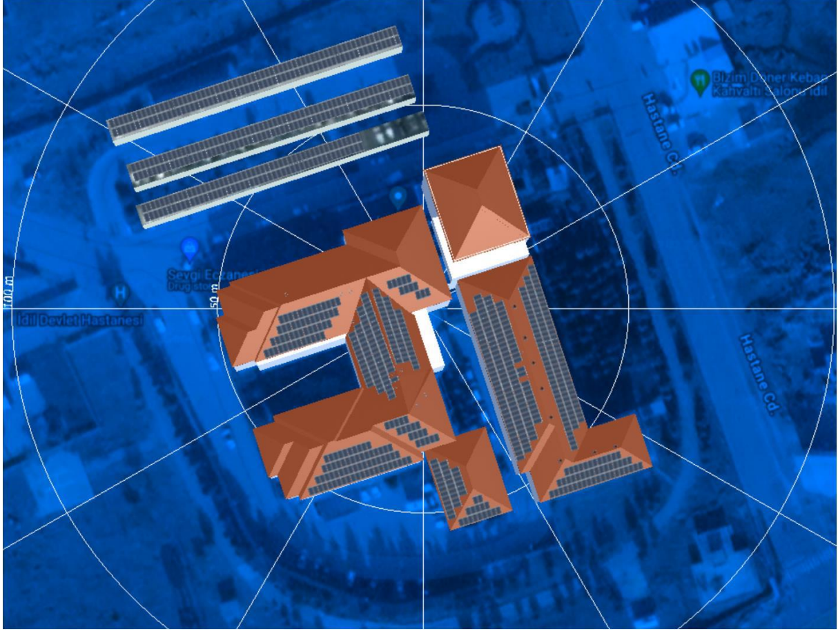
Şekil 4: Şırnak İdil Devlet Hastanesi Çatı ve Otopark Üstü PV Kurulum Tasarım Görünümü
